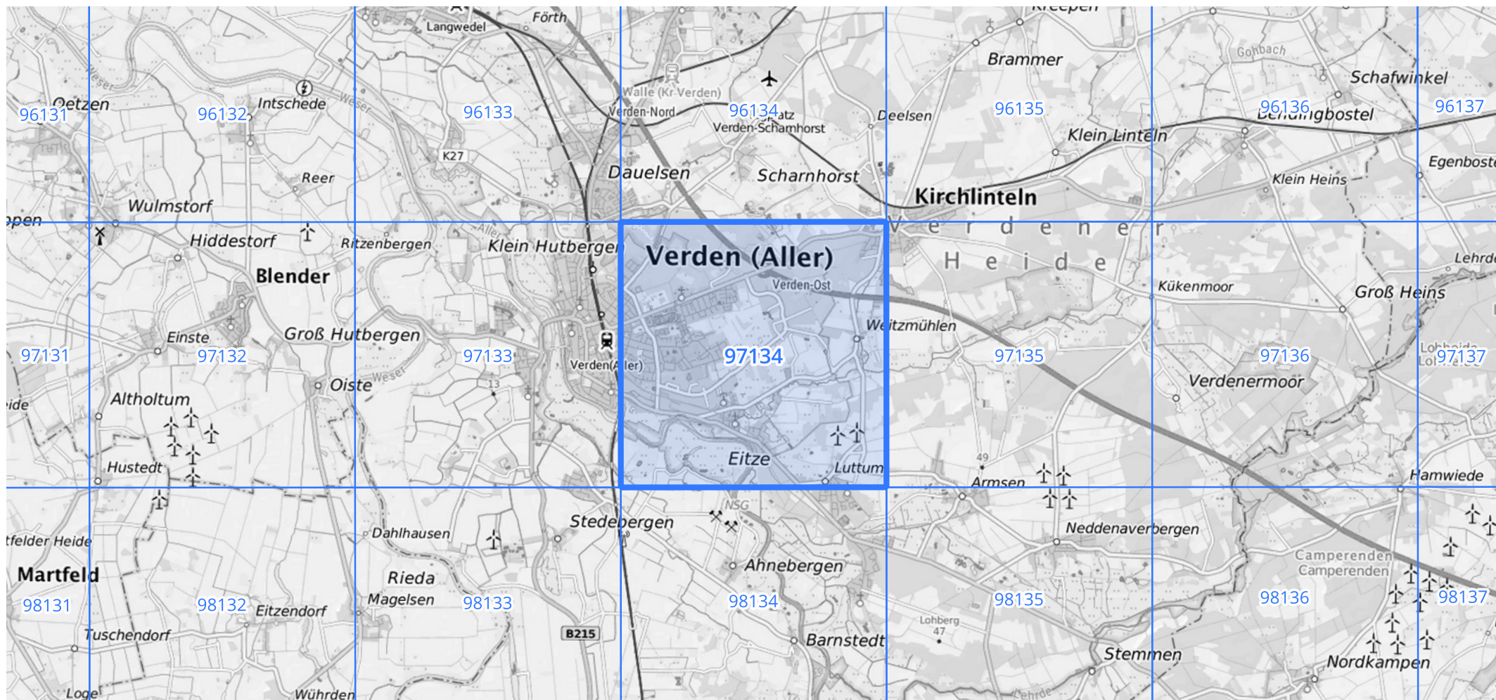
Übersichtskarte des Rasterfeldes 97134, M 1 : 100 000
