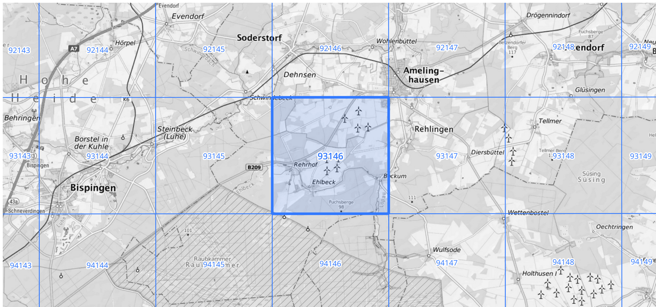
Übersichtskarte des Rasterfeldes 93146, M 1 : 100 000
