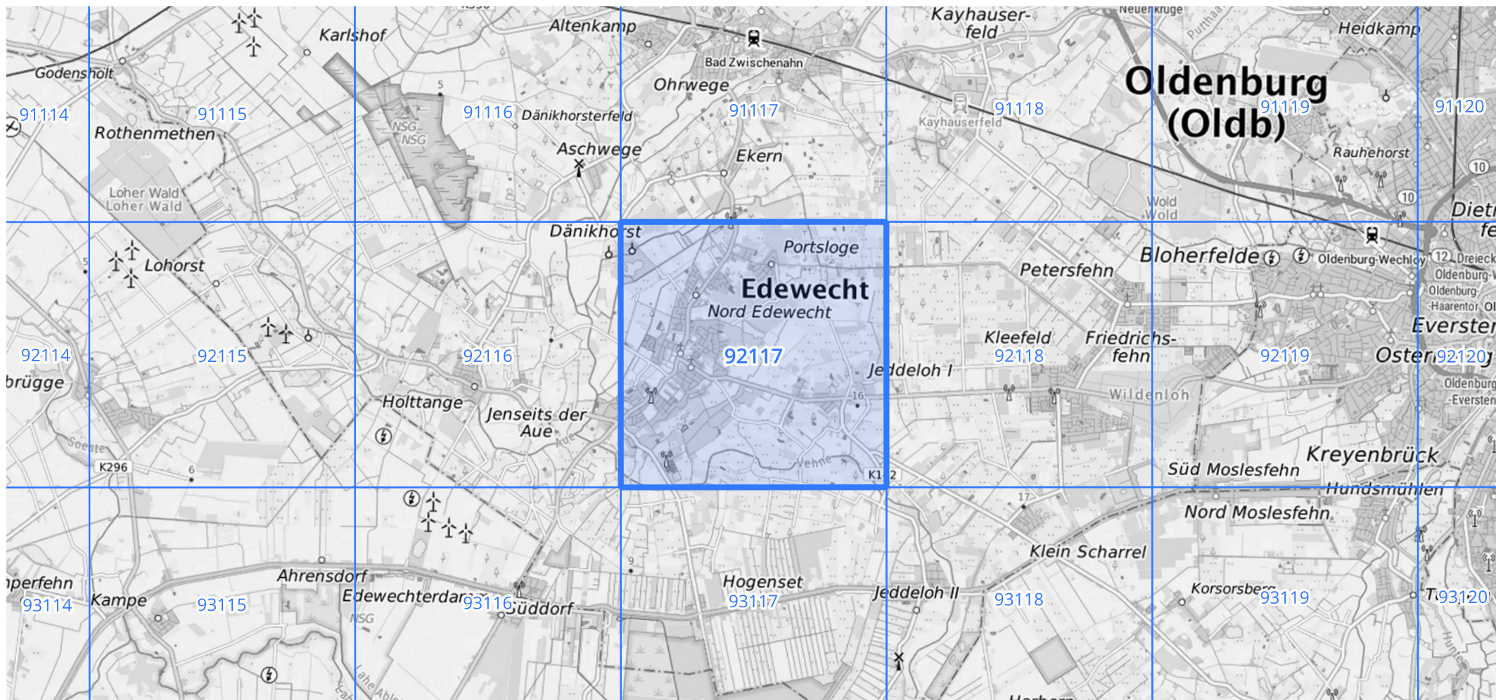
Übersichtskarte des Rasterfeldes 92117, M 1 : 100 000
