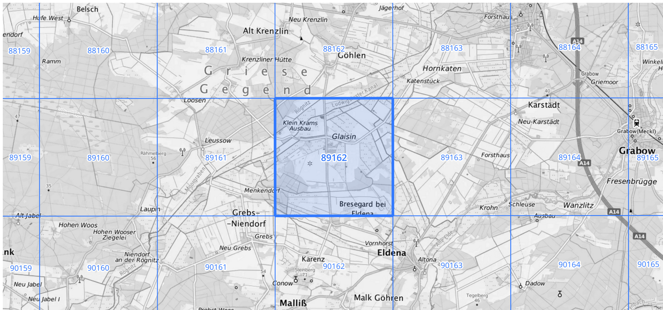
Übersichtskarte des Rasterfeldes 89162, M 1 : 100 000
