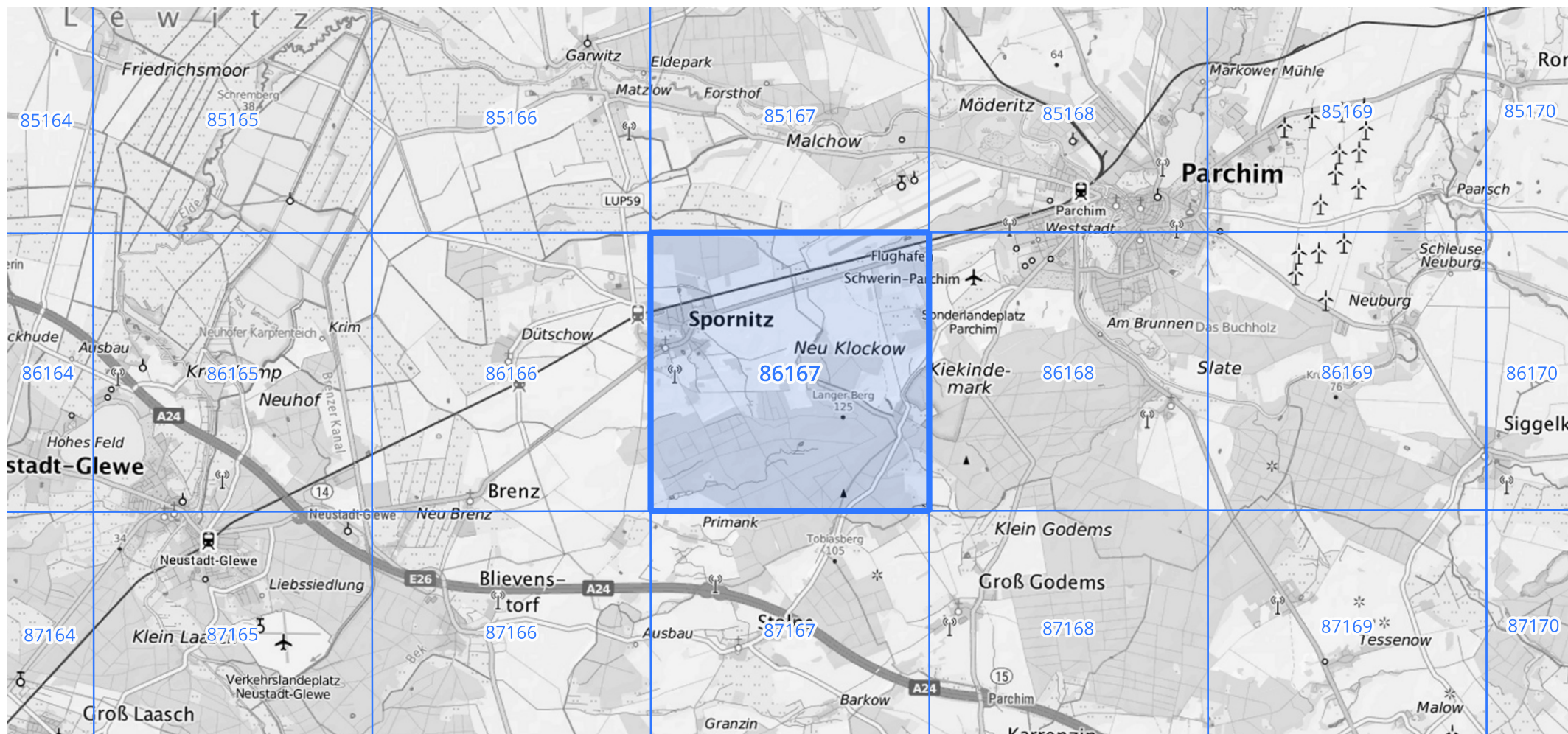
Übersichtskarte des Rasterfeldes 86167, M 1 : 100 000
