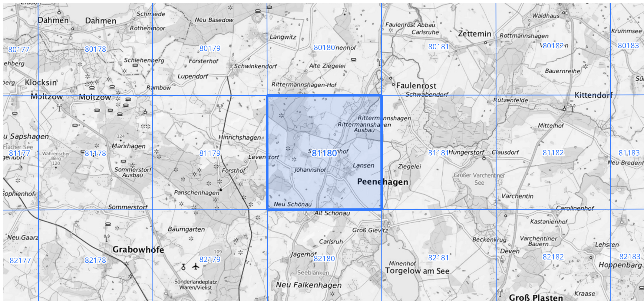
Übersichtskarte des Rasterfeldes 81180, M 1 : 100 000
