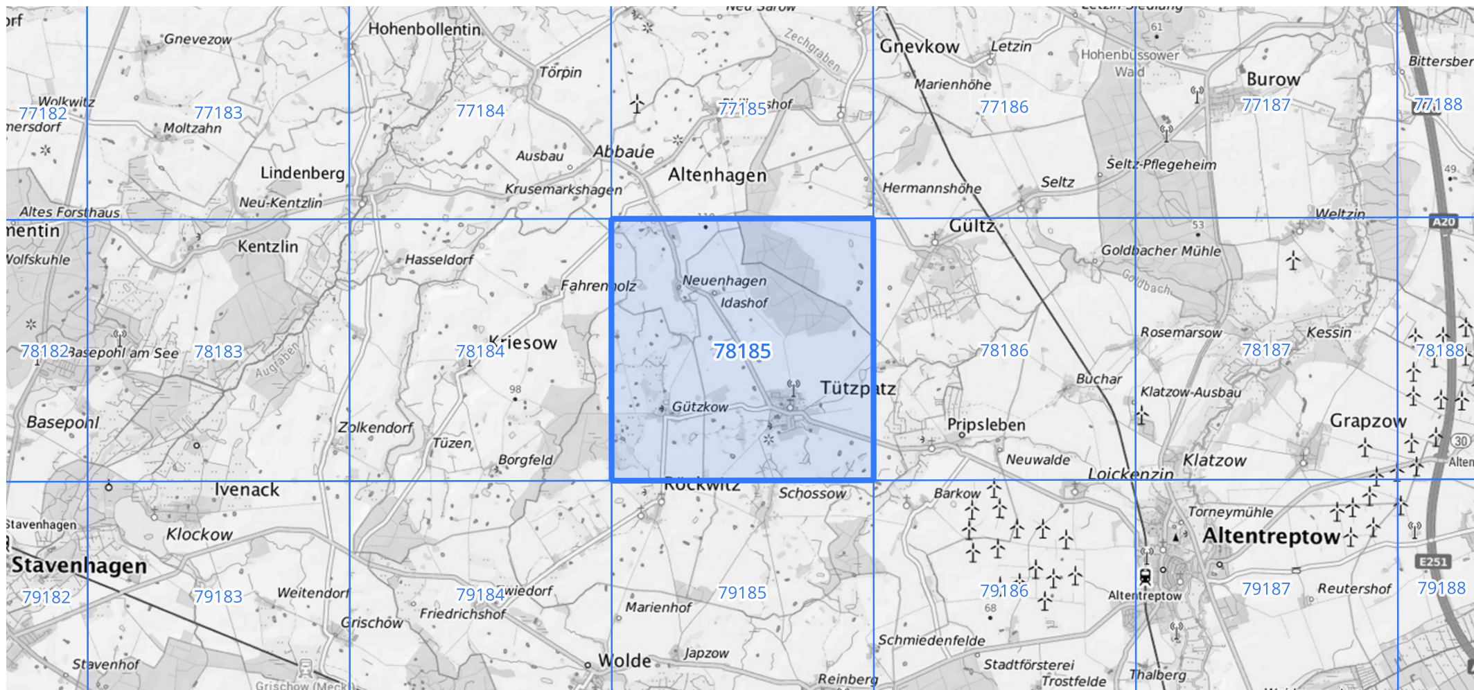
Übersichtskarte des Rasterfeldes 78185, M 1 : 100 000
