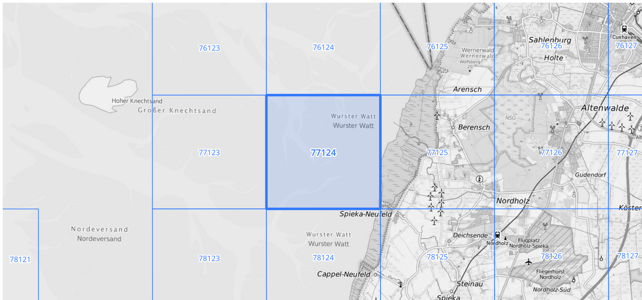
Übersichtskarte des Rasterfeldes 77124, M 1 : 100 000
