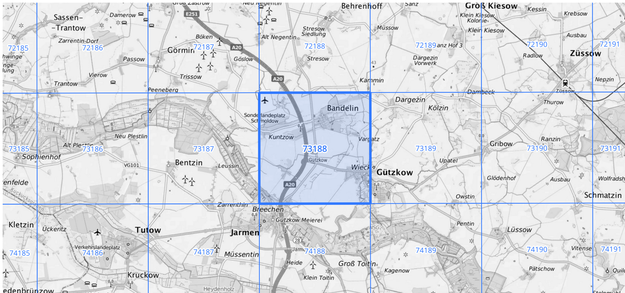
Übersichtskarte des Rasterfeldes 73188, M 1 : 100 000
