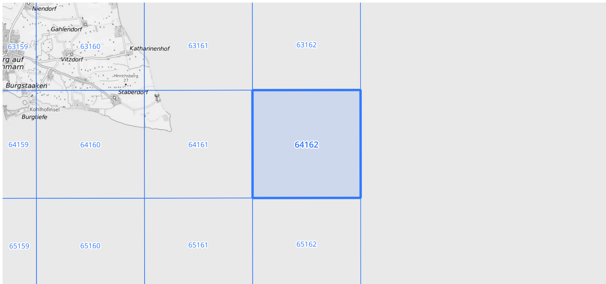
Übersichtskarte des Rasterfeldes 64162, M 1 : 100 000
