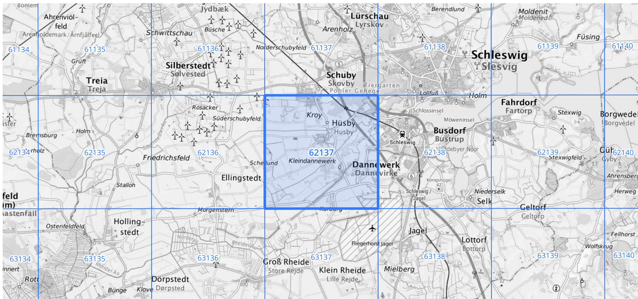
Übersichtskarte des Rasterfeldes 62137, M 1 : 100 000
