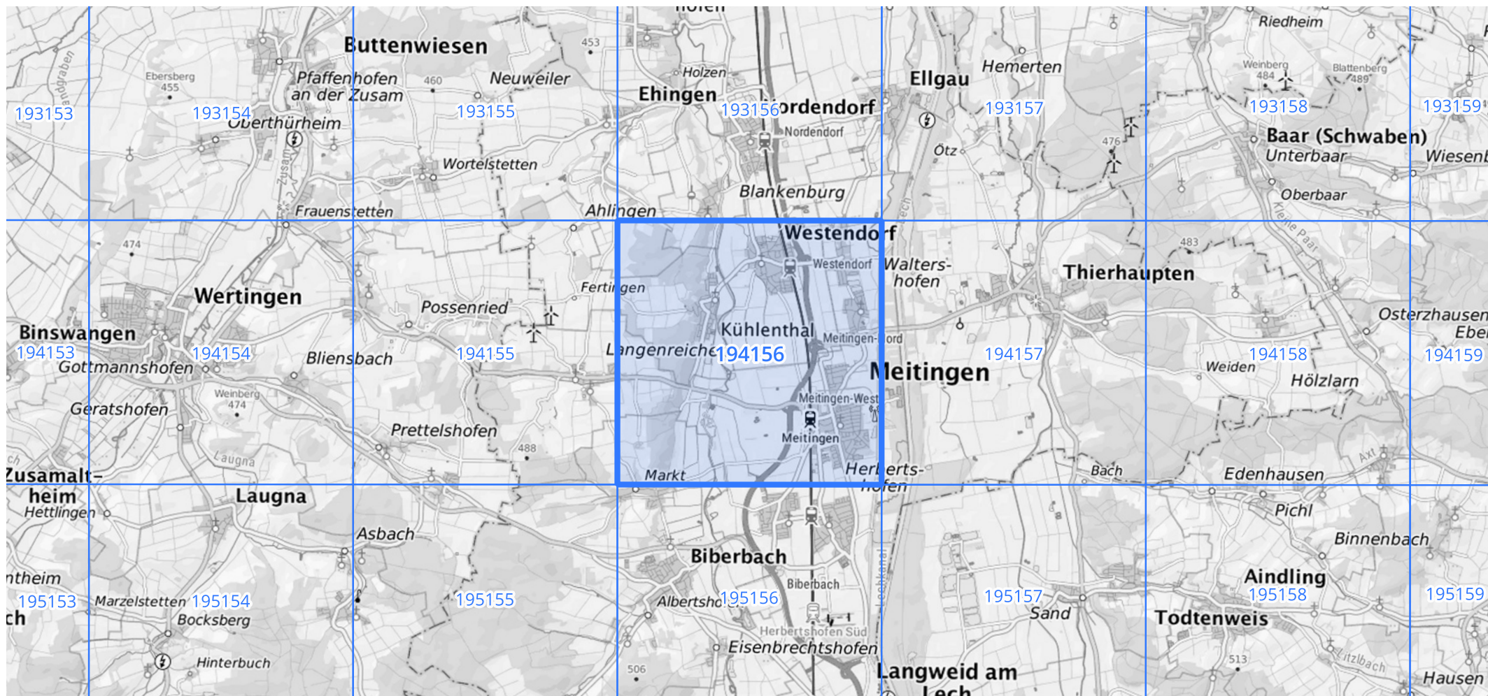
Übersichtskarte des Rasterfeldes 194156, M 1 : 100 000
