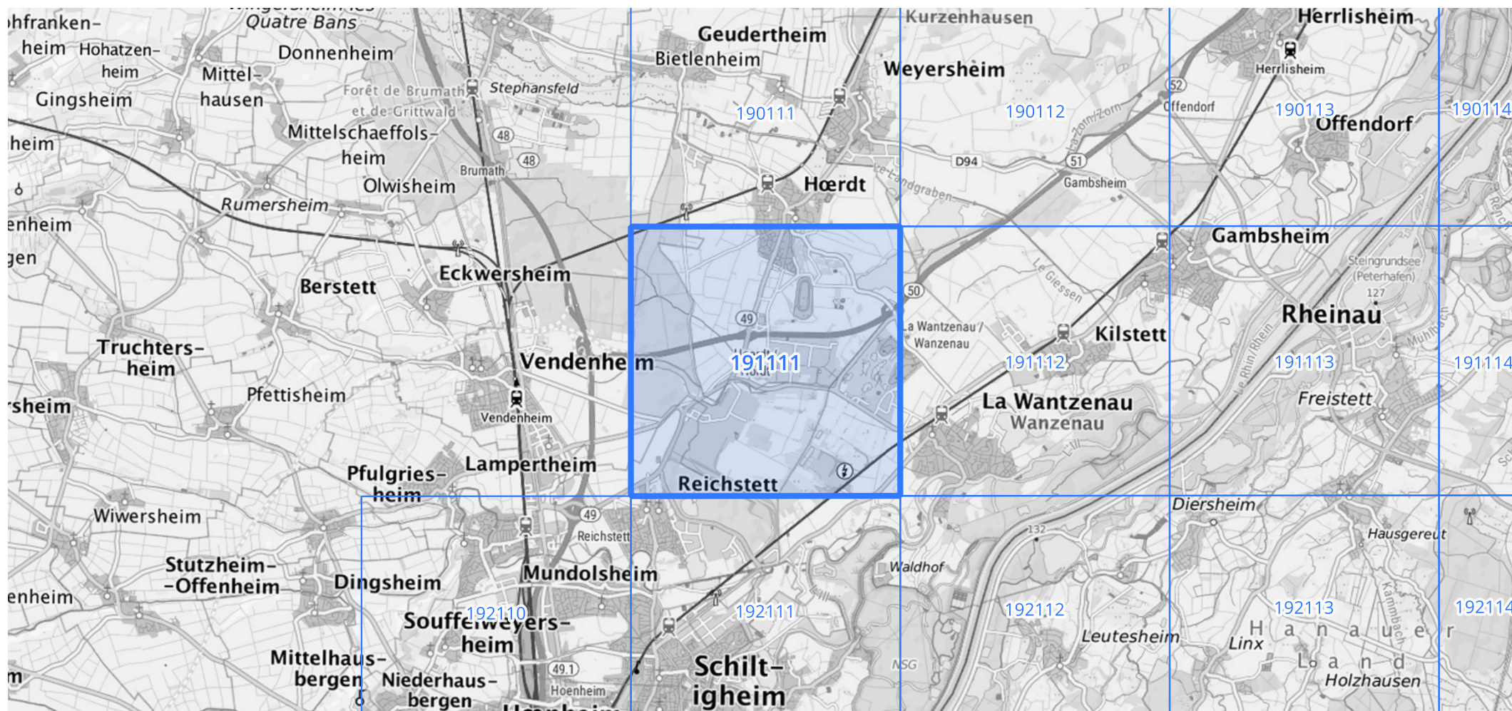
Übersichtskarte des Rasterfeldes 191111, M 1 : 100 000
