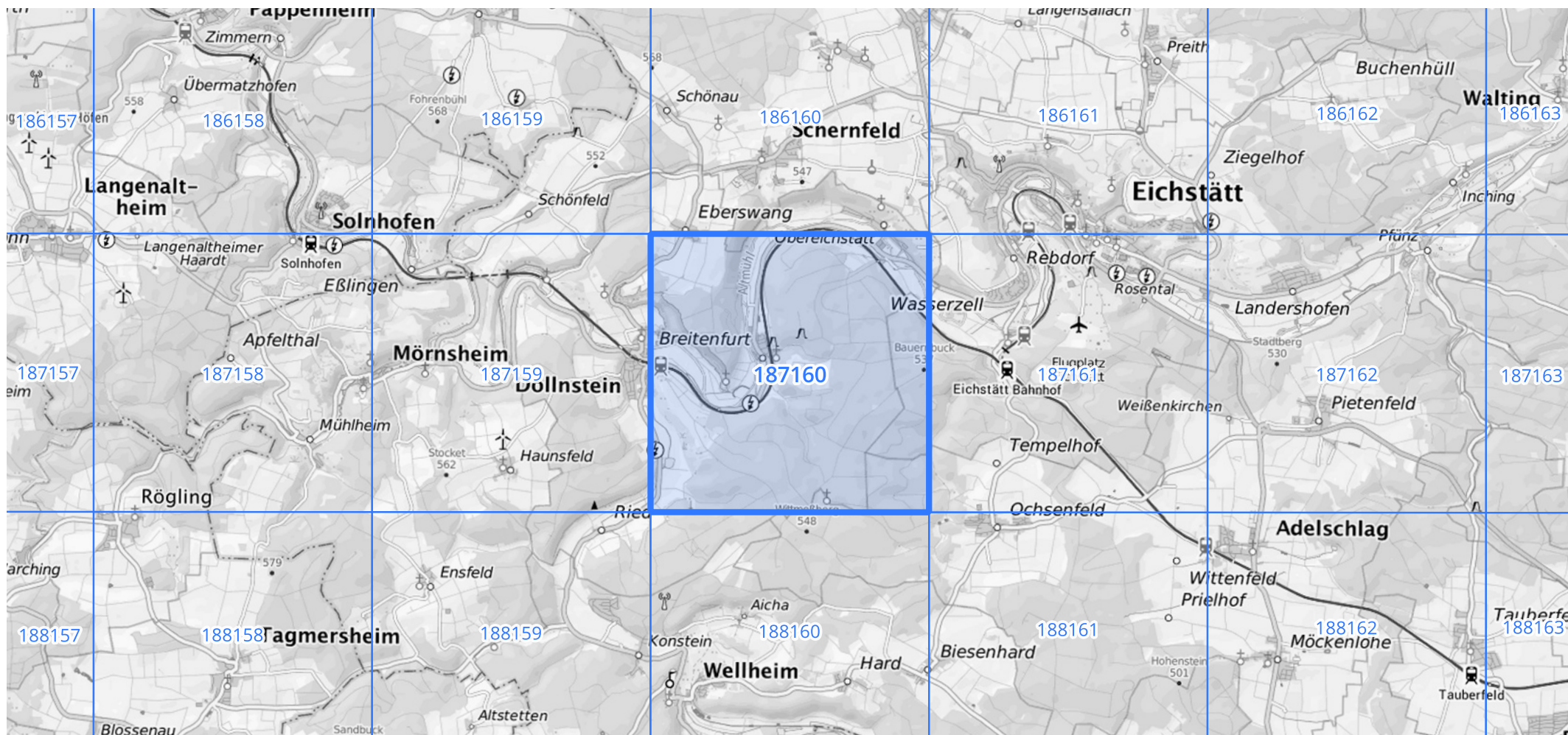
Übersichtskarte des Rasterfeldes 187160, M 1 : 100 000
