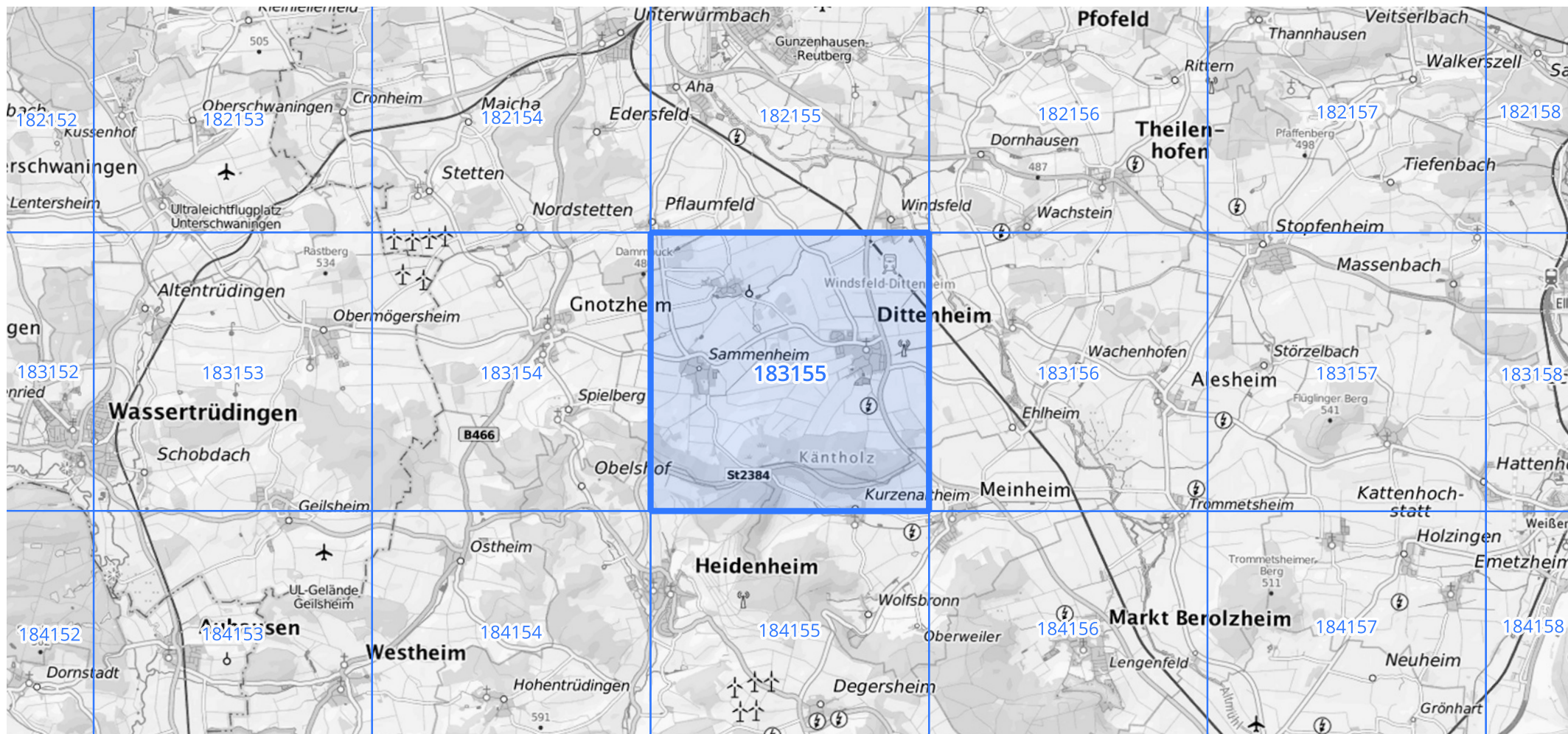
Übersichtskarte des Rasterfeldes 183155, M 1 : 100 000
