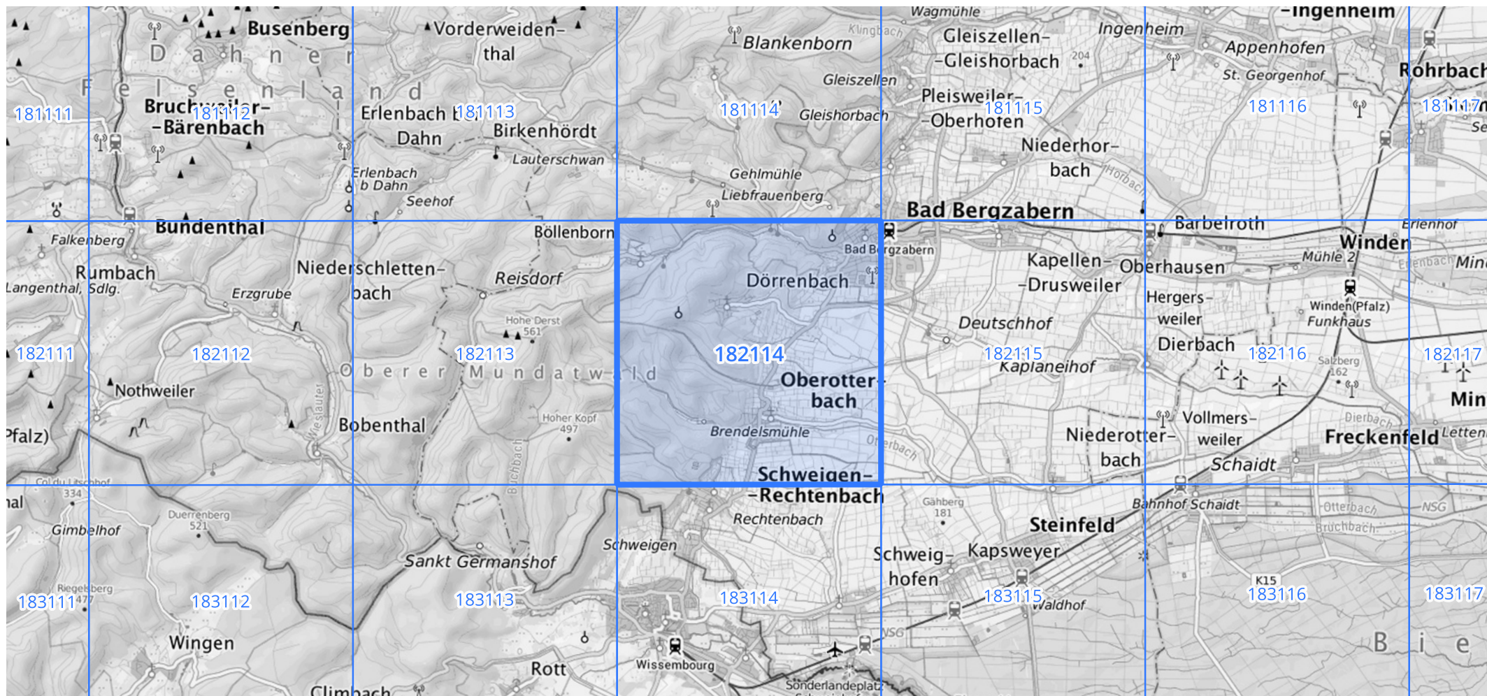
Übersichtskarte des Rasterfeldes 182114, M 1 : 100 000
