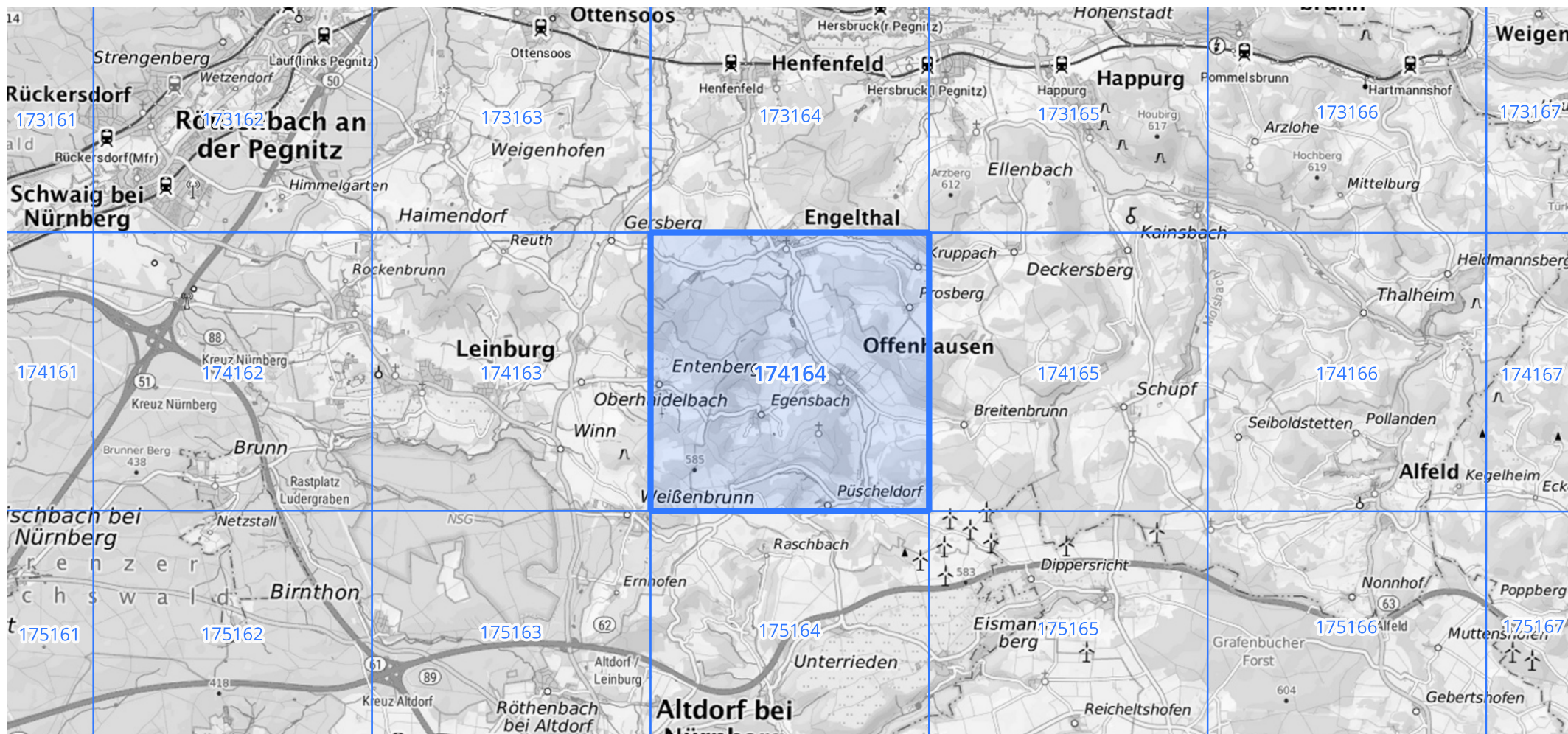
Übersichtskarte des Rasterfeldes 174164, M 1 : 100 000
