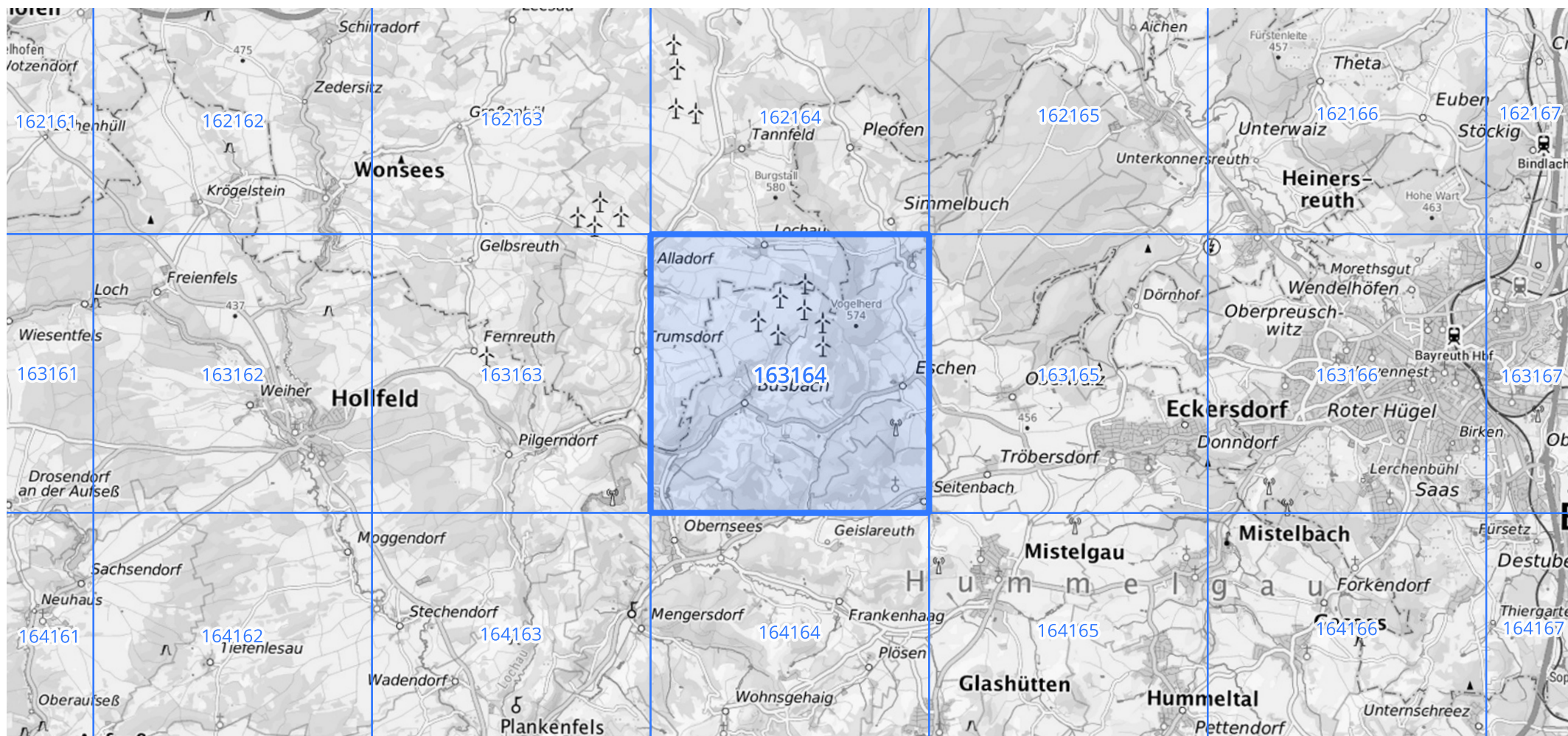
Übersichtskarte des Rasterfeldes 163164, M 1 : 100 000
