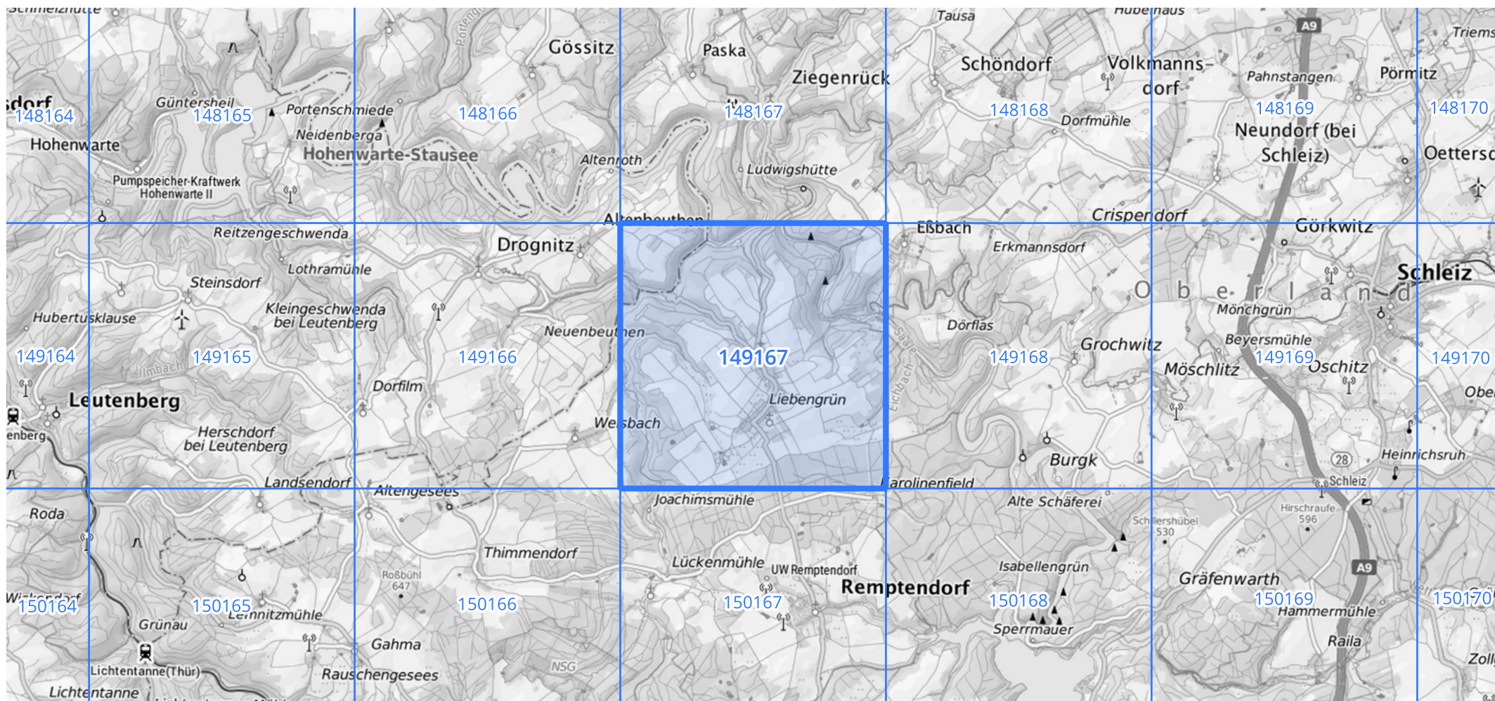
Übersichtskarte des Rasterfeldes 149167, M 1 : 100 000
