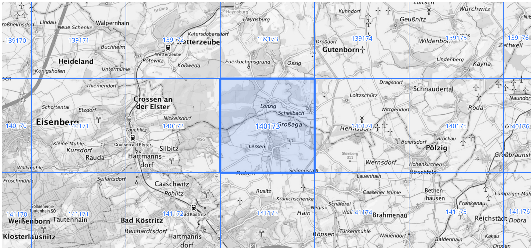
Übersichtskarte des Rasterfeldes 140173, M 1 : 100 000
