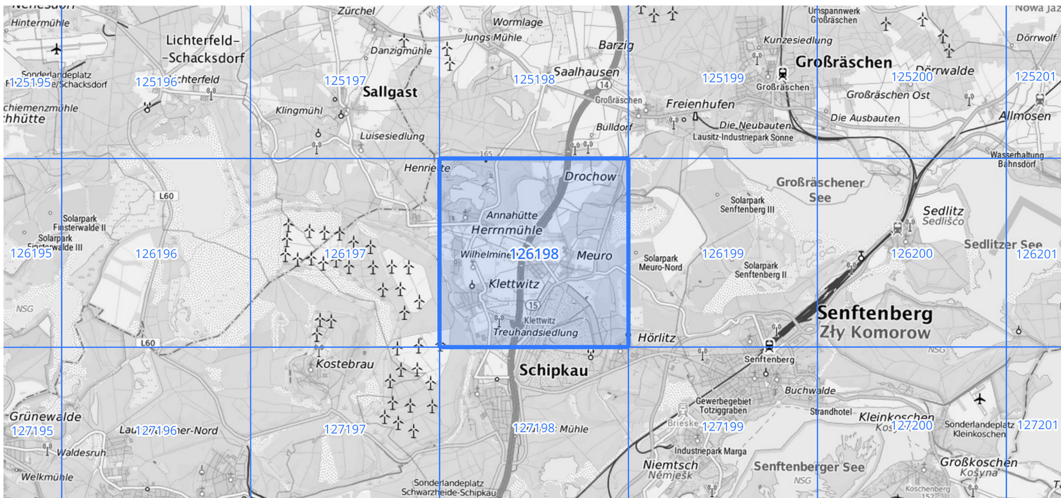
Übersichtskarte des Rasterfeldes 126198, M 1 : 100 000
