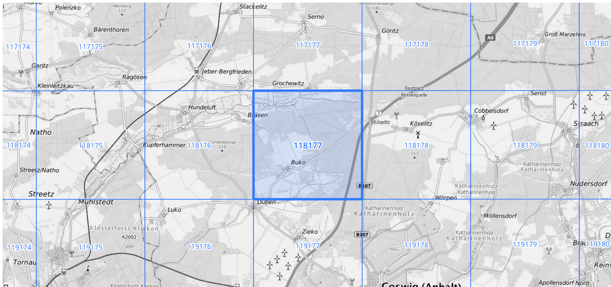
Übersichtskarte des Rasterfeldes 118177, M 1 : 100 000
