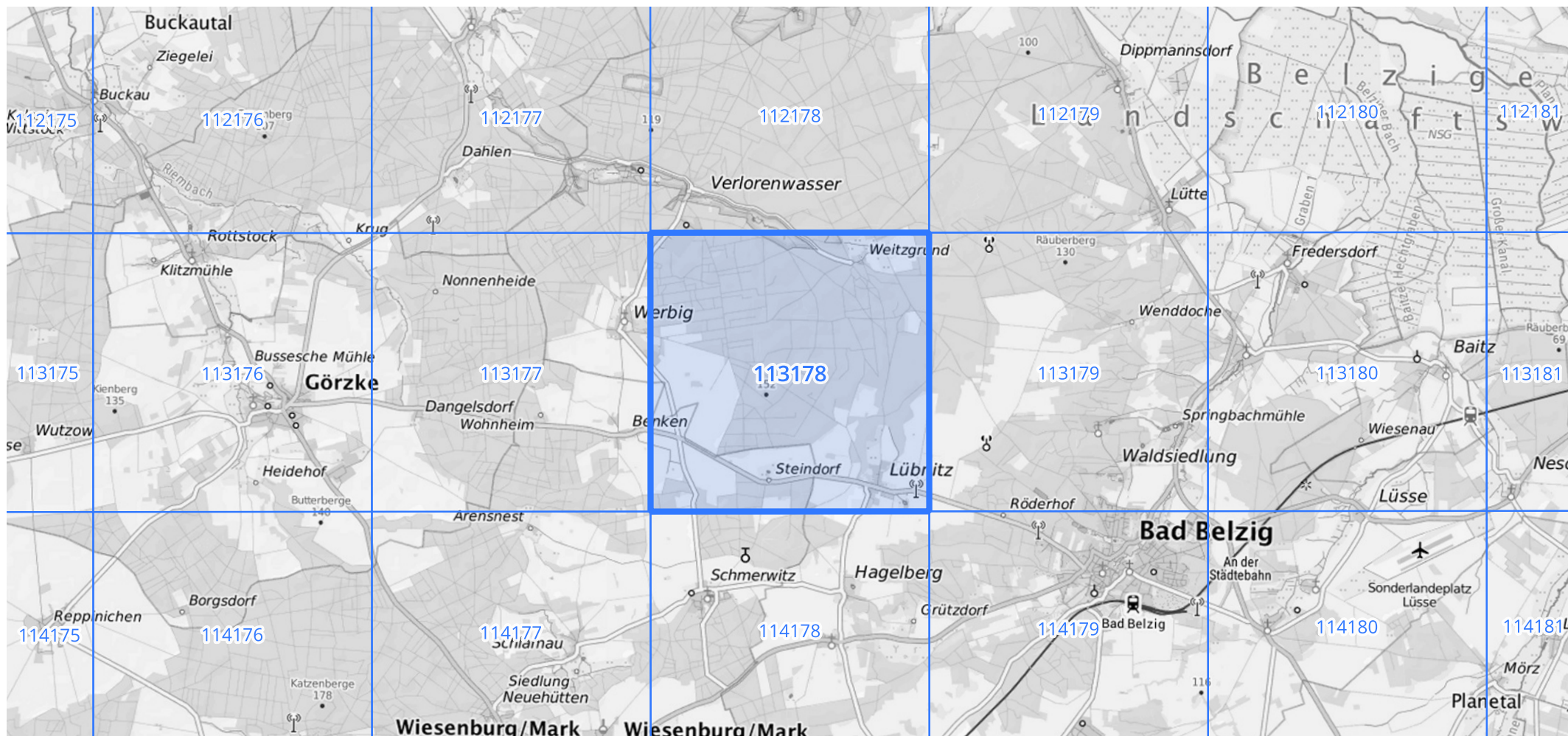
Übersichtskarte des Rasterfeldes 113178, M 1 : 100 000
