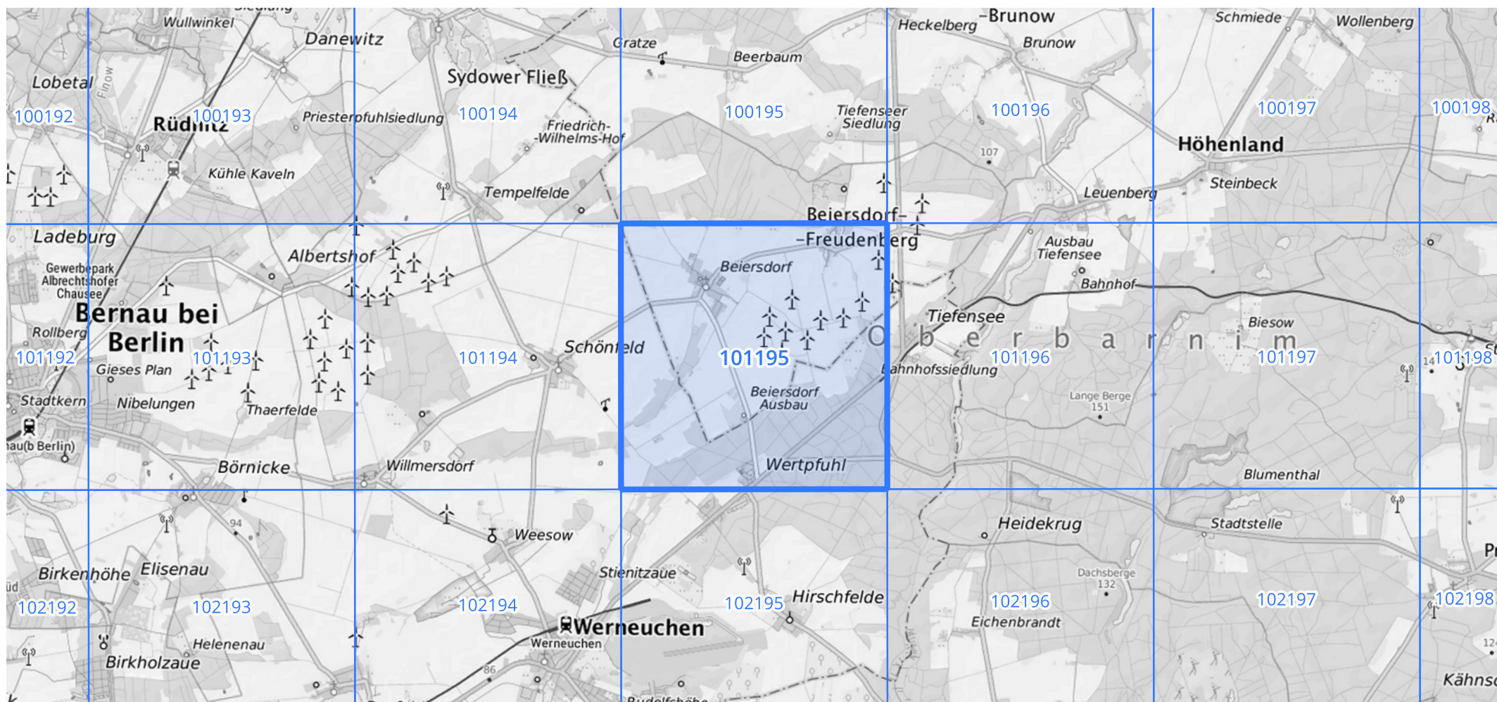
Übersichtskarte des Rasterfeldes 101195, M 1 : 100 000
